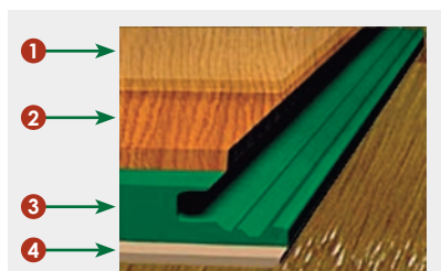
Coupe d'une lame de parquet contrecollé
